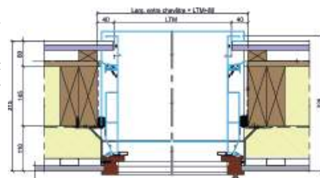
COUPE HORIZONTALE
