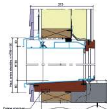
COUPE VERTICALE
