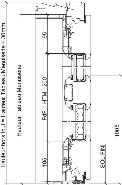
coupe verticale
