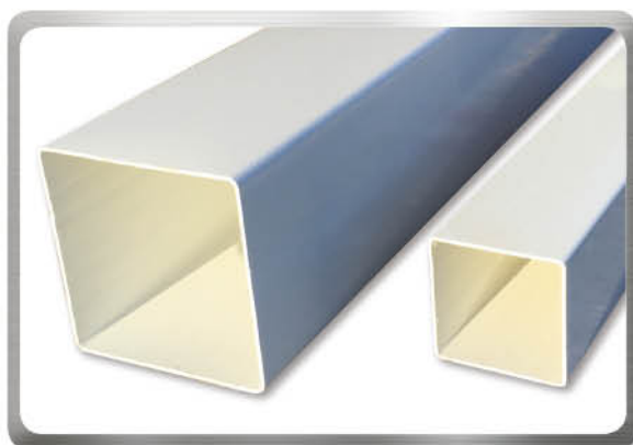
Poteau PVC 120 x 120 scellement de 500 mm Poteau PVC 200 x 200 scellement de 500 mm
