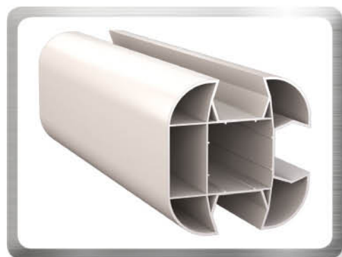
Poteau clôture PVC Éco 96 x 96 Poteau 96 X 96 mm avec platine acier à visser
