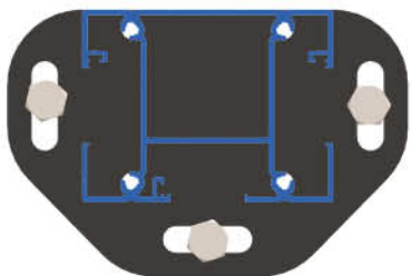
Poteau alu 84 X 64 mm, avec platine
